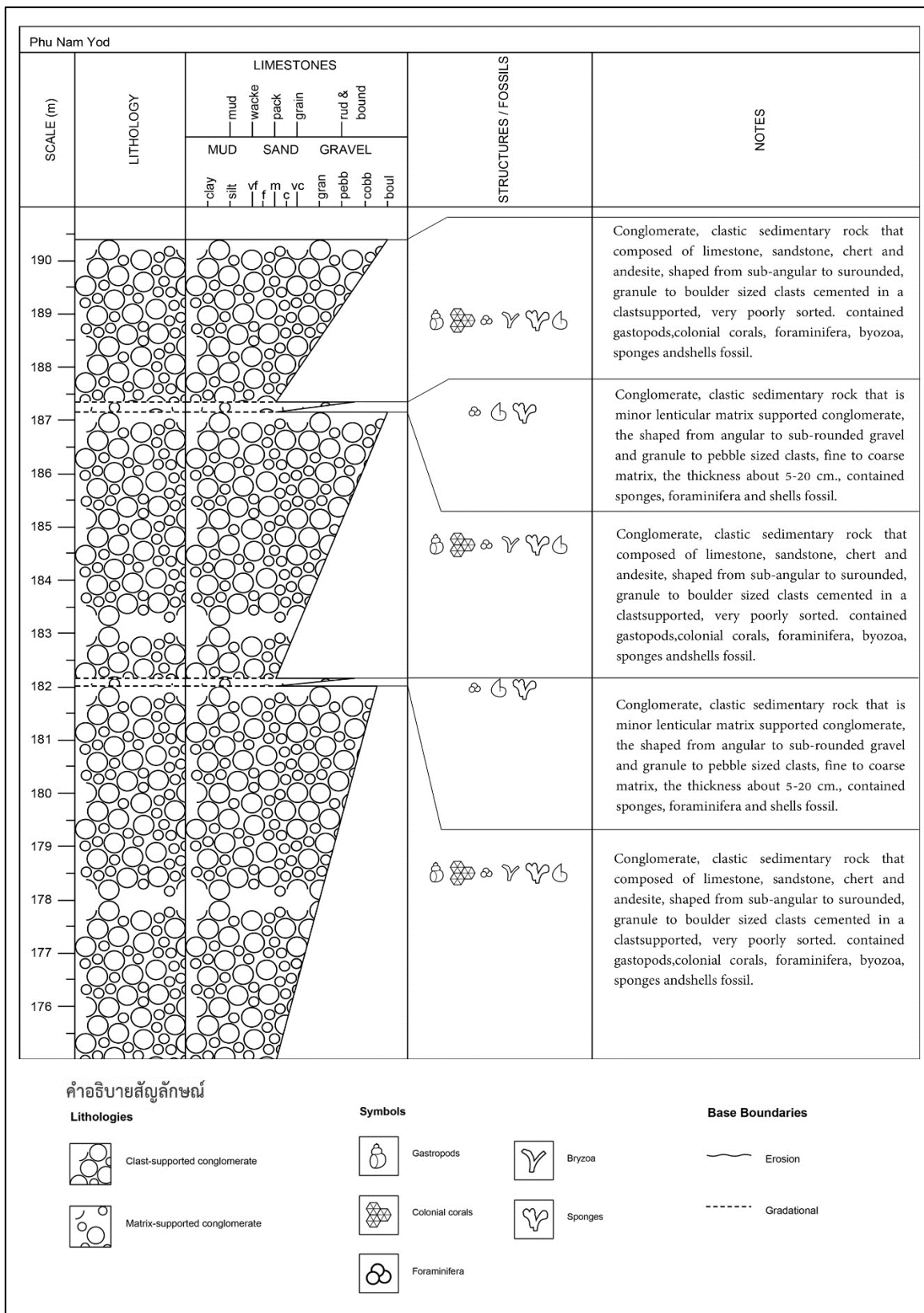
รูปที่ ๒.๕ ลำดับชั้นหินในพื้นที่แหล่งซากดึกดำบรรพ์สัตว์ไม่มีกระดูกสันหลังภูน้ำหยด
