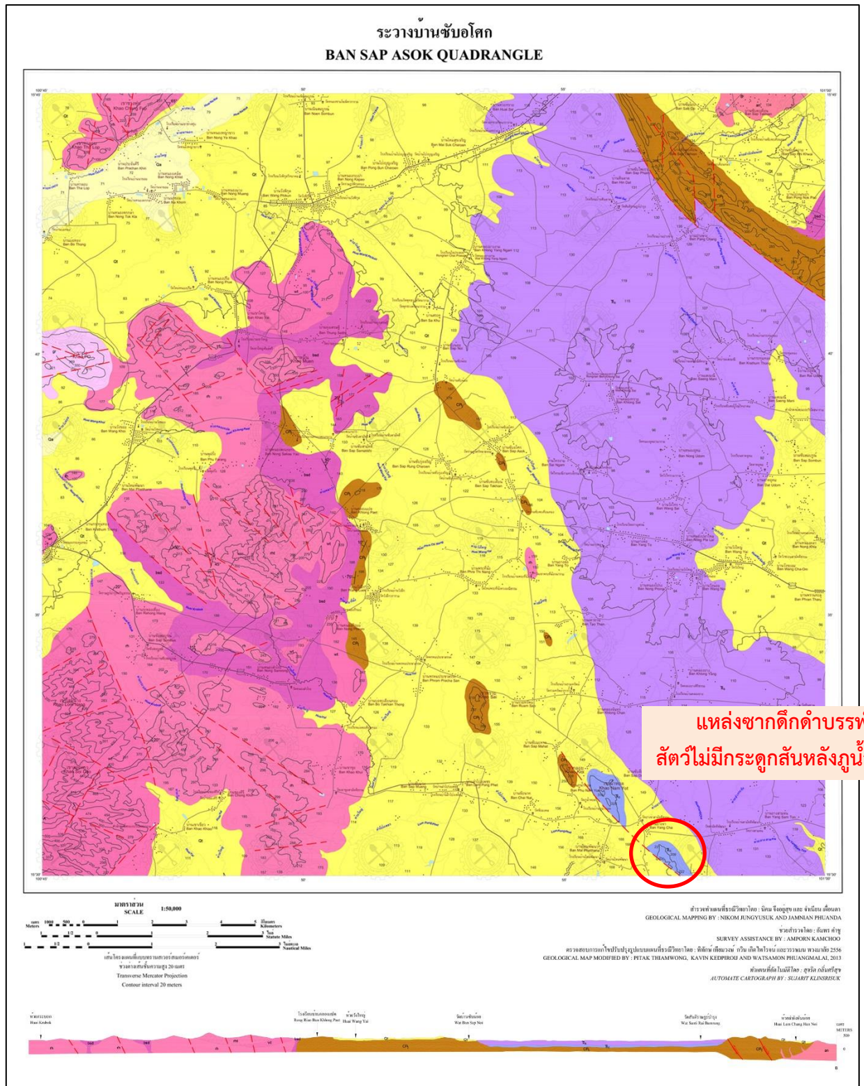
รูปที่ ๒.๔ แผนที่ธรณีวิทยา ระวางบ้านซ้อโตก (๕๑๐๔ II) มาตรฐาน ๑ : ๕๐,๐๐๐ (กรมทรัพยากรธรณี, ๒๕๕๖)
