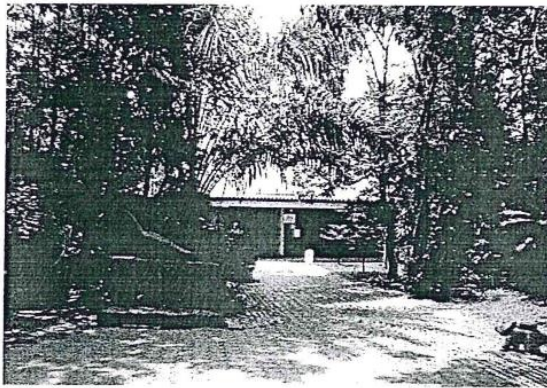
รูปถ่ายอาคารคลุมแหล่งซากไดโนเสาร์ภูมู่ข้าว จังหวัดกาฬสินธุ์
