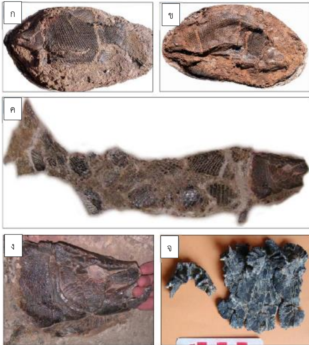
รูปที่ ๒.๕ ซากดึกดำบรรพ์ปลาโบราณที่พบบริเวณแหล่งปลาโบราณภูน้ำจั้น
