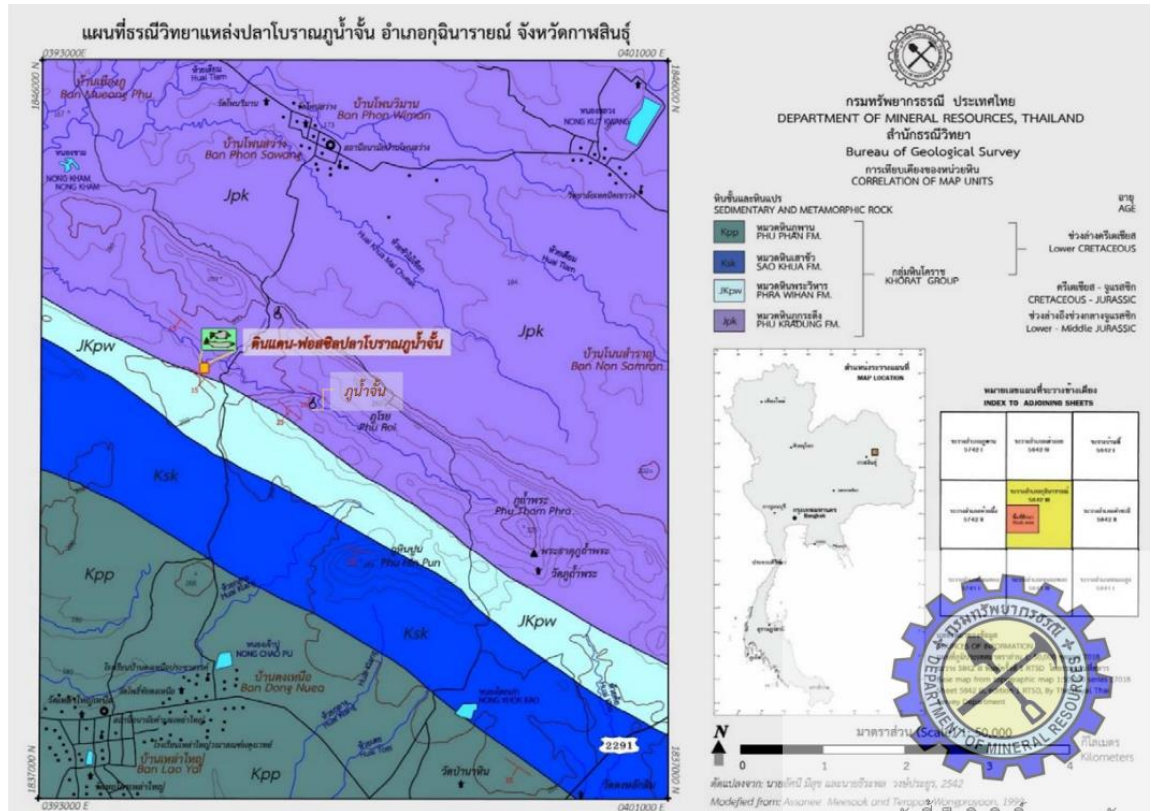
รูปที่ ๒.๔ แผนที่ธรณีวิทยาบริเวณภูน้ำจั้น (วารุณี ยะถากรรม และกิตติ ขาววิเศษ, ๒๕๖๐)
