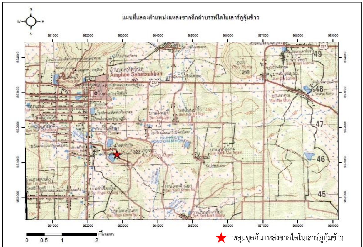
รูปที่ ๒.๑๓ แหล่งซากไดโนเสาร์ภูกุ่มข้าว
