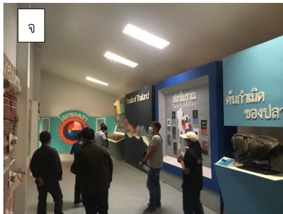
รูปที่ ๒.๗ แหล่งปลาโบราณภูน้ำจั้น จังหวัดกาฬสินธุ์
