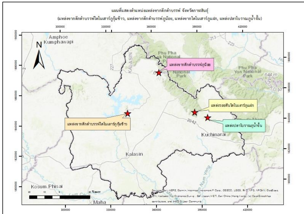
รูปที่ ๑.๑ แสดงตำแหน่งแหล่งซากดึกดำบรรพ์ที่ขึ้นทะเบียน แหล่งปลาโบราณน้ำจืด แหล่งรอยตีนไดโนเสาร์ภูแฝก แหล่งซากไดโนเสาร์ภูกุ่มข้าว และแหล่งซากดึกดำบรรพ์ภูน้อย จังหวัดกาฬสินธุ์
