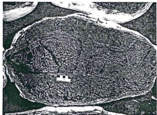
รูปถ่ายซากปลาโบราณที่อยู่ในแหล่งปลาโบราณภูน้ำจั้น จังหวัดกาฬสินธุ์
