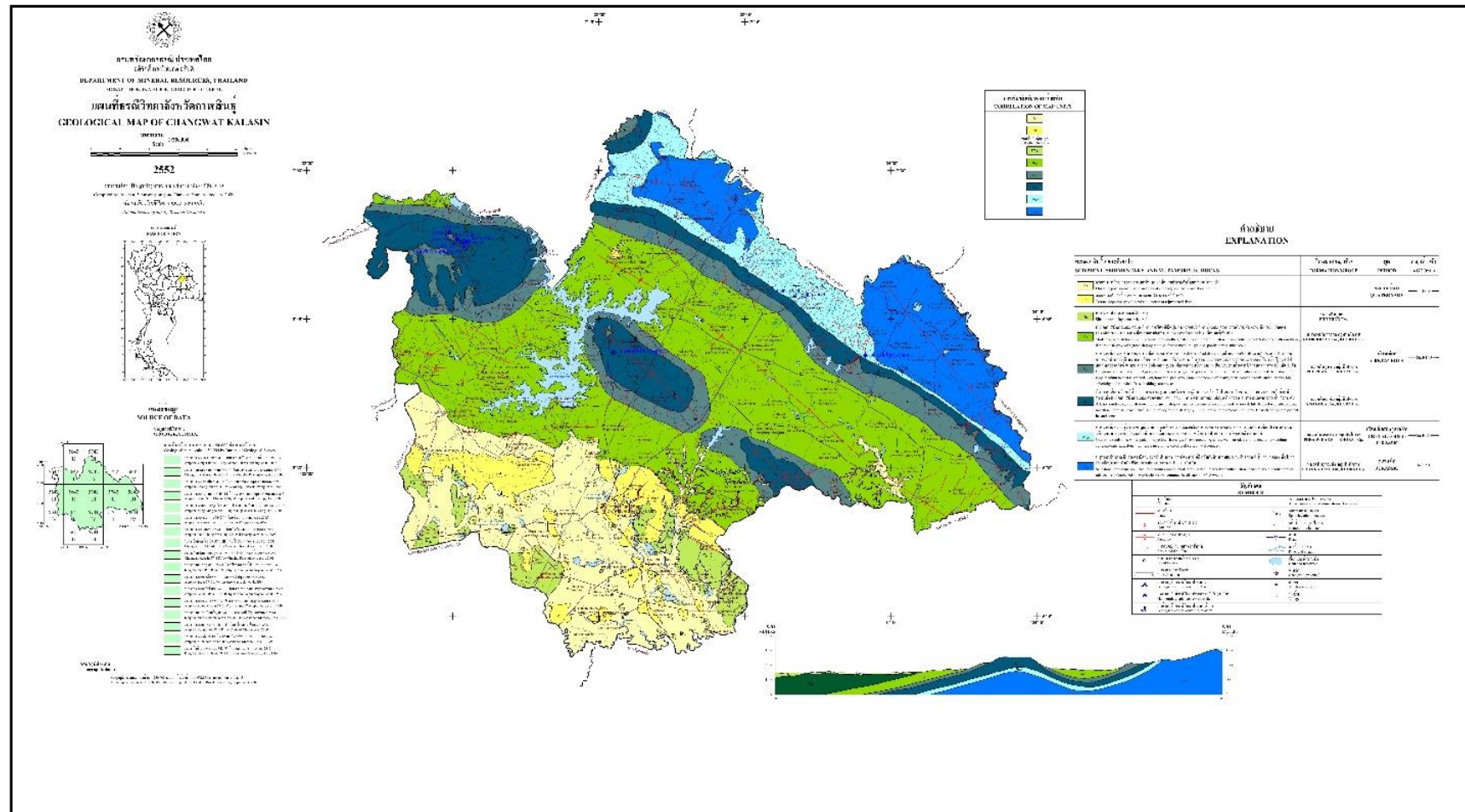
รูปที่ ๒.๒ แผนที่ธรณีวิทยาจังหวัดกาฬสินธุ์ (กรมทรัพยากรธรณี, ๒๕๕๒)
