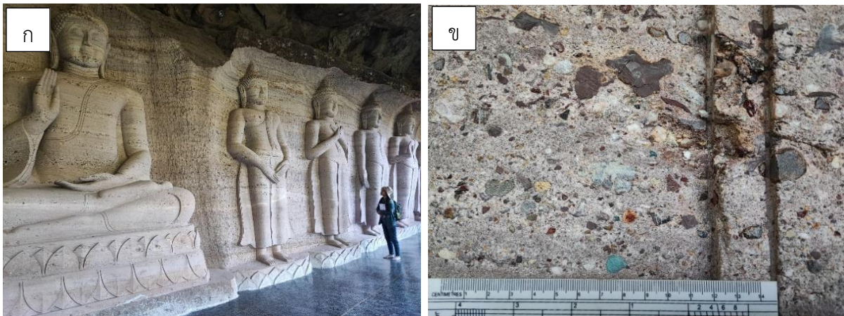
รูปที่ ๒.๓๐ แหล่งธรณีสัณฐานภูตนาไห (ก) ลักษณะประติมากรรมแกะสลักพระพุทธรูปในหมวดหินภูพาน บริเวณสำนักสงฆ์ (ข) ลักษณะของเนื้อหิน (โชติมา ยามี่ และคณะ, ๒๕๖๖)
