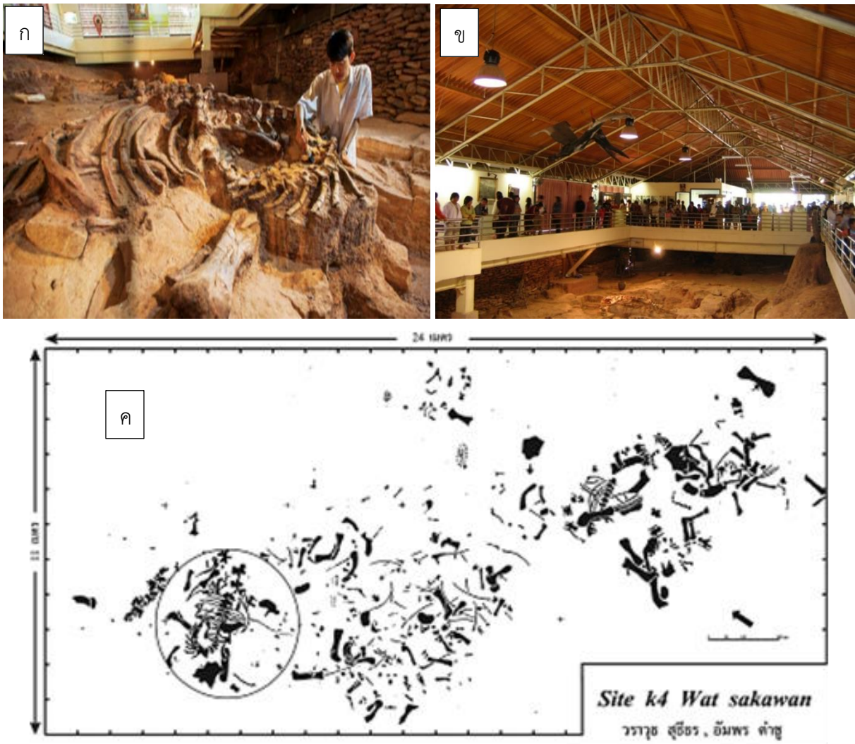
รูปที่ ๒.๑๖ แหล่งซากไดโนเสาร์ภูมู่ข้าว
