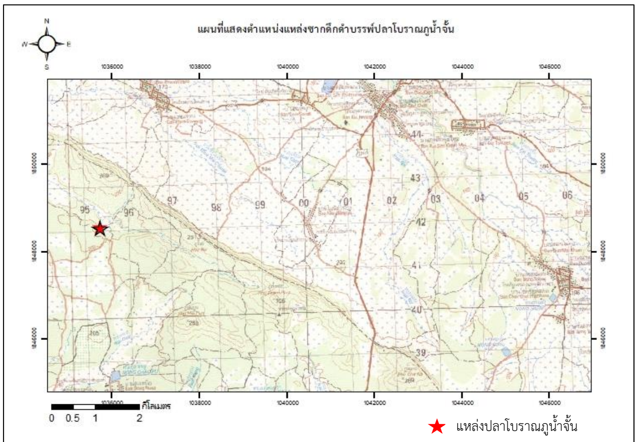
รูปที่ ๒.๓ แผนที่แสดงตำแหน่งแหล่งปลาโบราณภูน้ำจั้น
