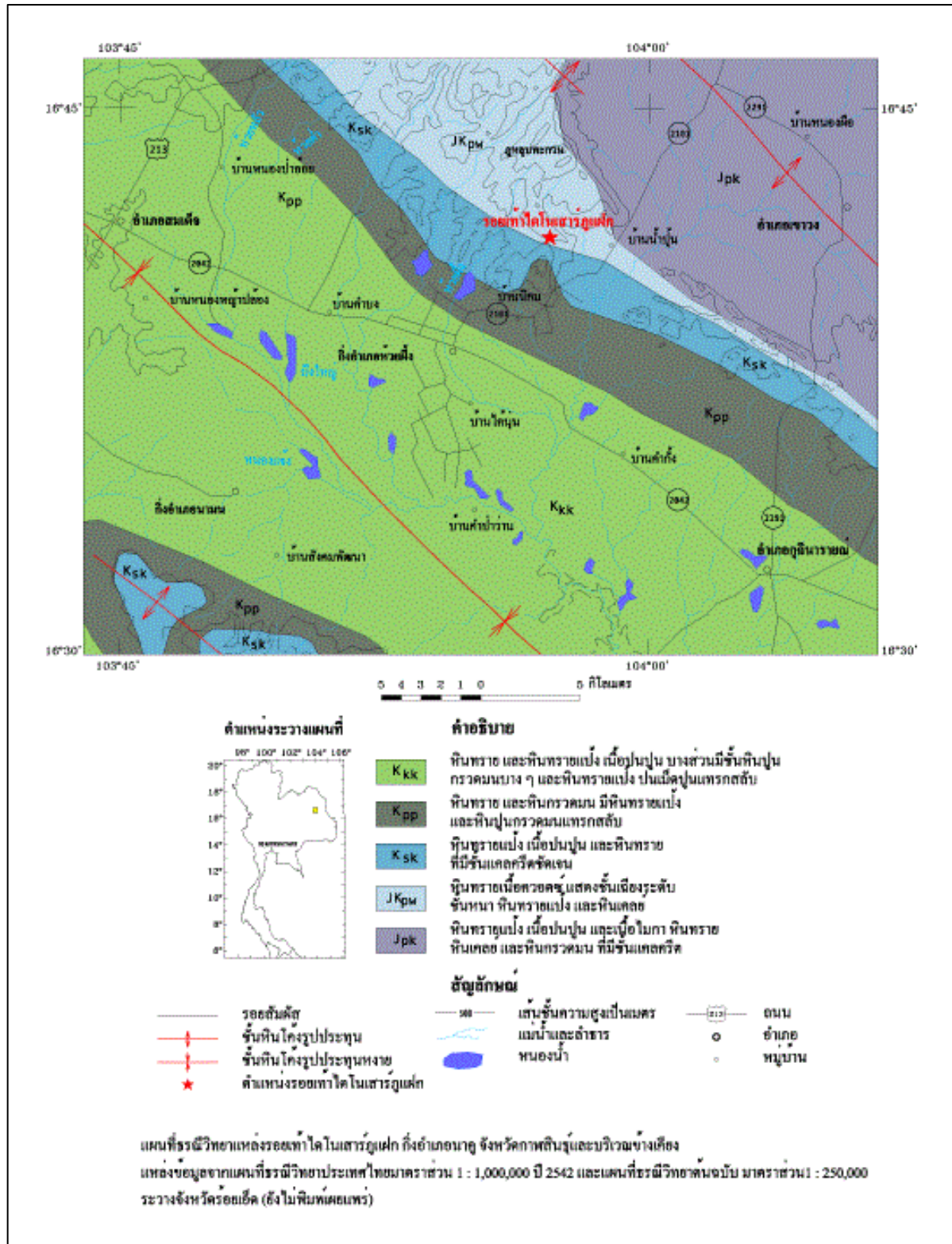
รูปที่ ๒.๙ แผนที่ธรณีวิทยาบริเวณแหล่งรอยตีนไดโนเสาร์ภูผาเหล็ก
