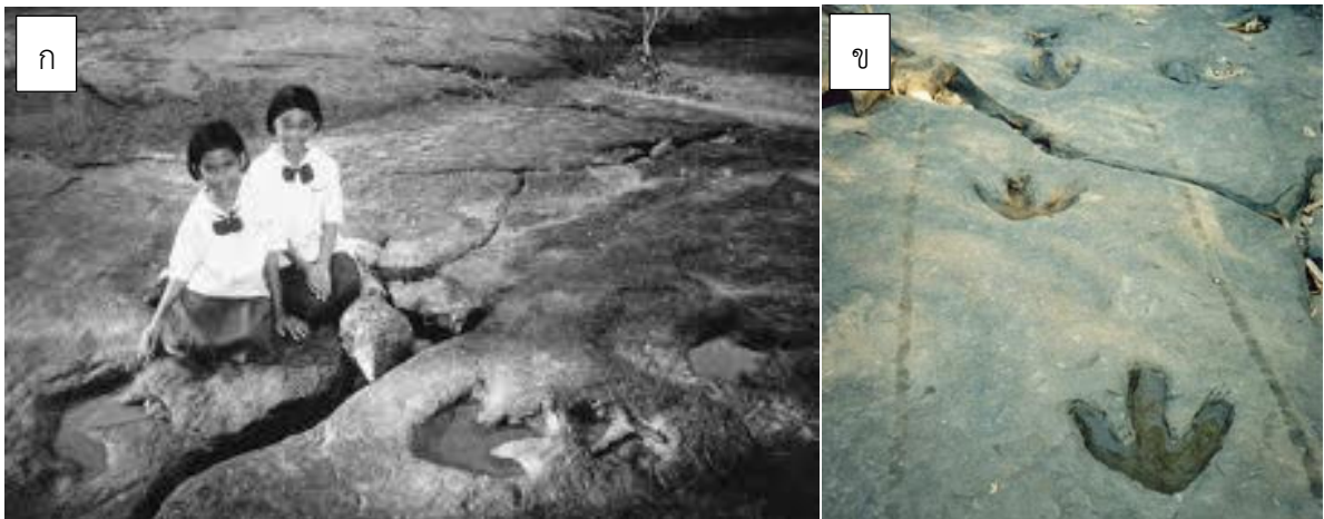
รูปที่ ๒.๑๐ รอยตีนไดโนเสาร์ที่พบในลำห้วยพะยังบริเวณภูแฝก
