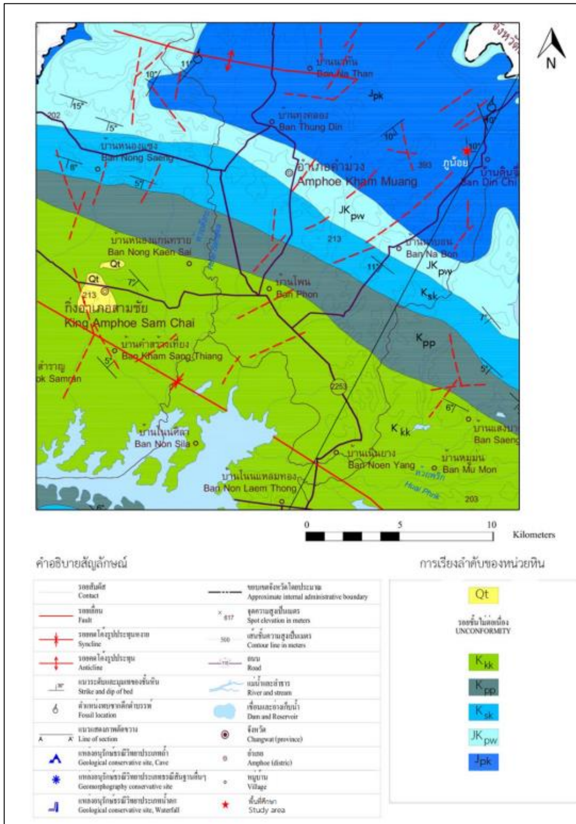
รูปที่ ๒.๑๘ แผนที่ธรณีวิทยา พื้นที่แหล่งซากดึกดำบรรพ์ภูน้อย (พรเพ็ญ จันทสิทธิ์และคณะ, ๒๕๖๐)
