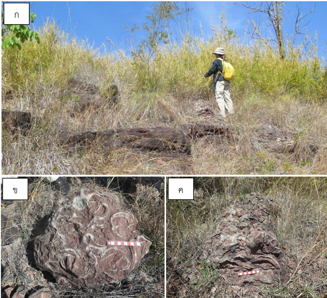
รูปที่ ๒.๒๓ แหล่งซากดึกดำบรรพ์สุสานหอยภูสิงห์
