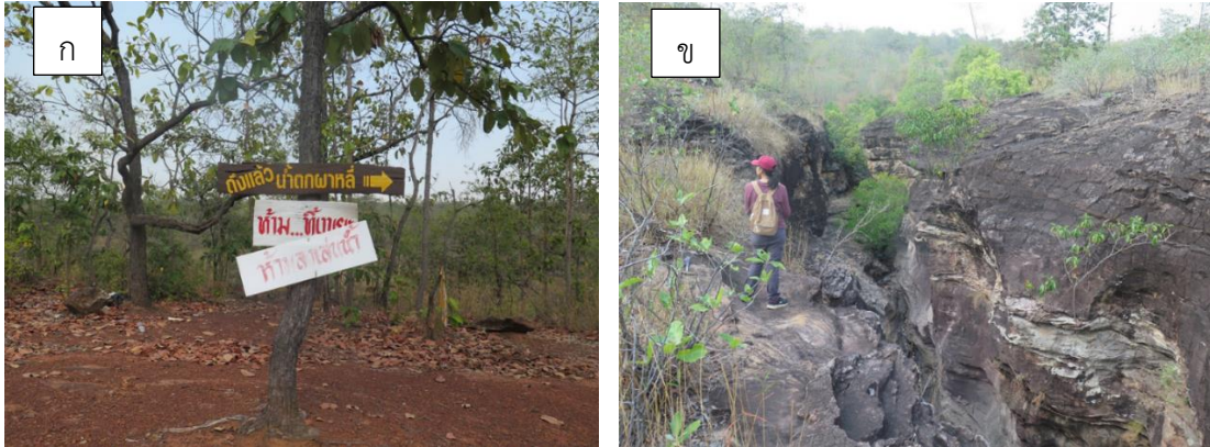
รูปที่ ๒.๒๘ แหล่งธรณีสัณฐานน้ำตกผาลี่ (ก) ป้ายทางเข้าน้ำตกผาลี่ (ผาลี่) และ (ข) ลักษณะน้ำตกผาลี่ ในฤดูแล้ง (โชติมา ยามิ และคณะ, ๒๕๖๖)
