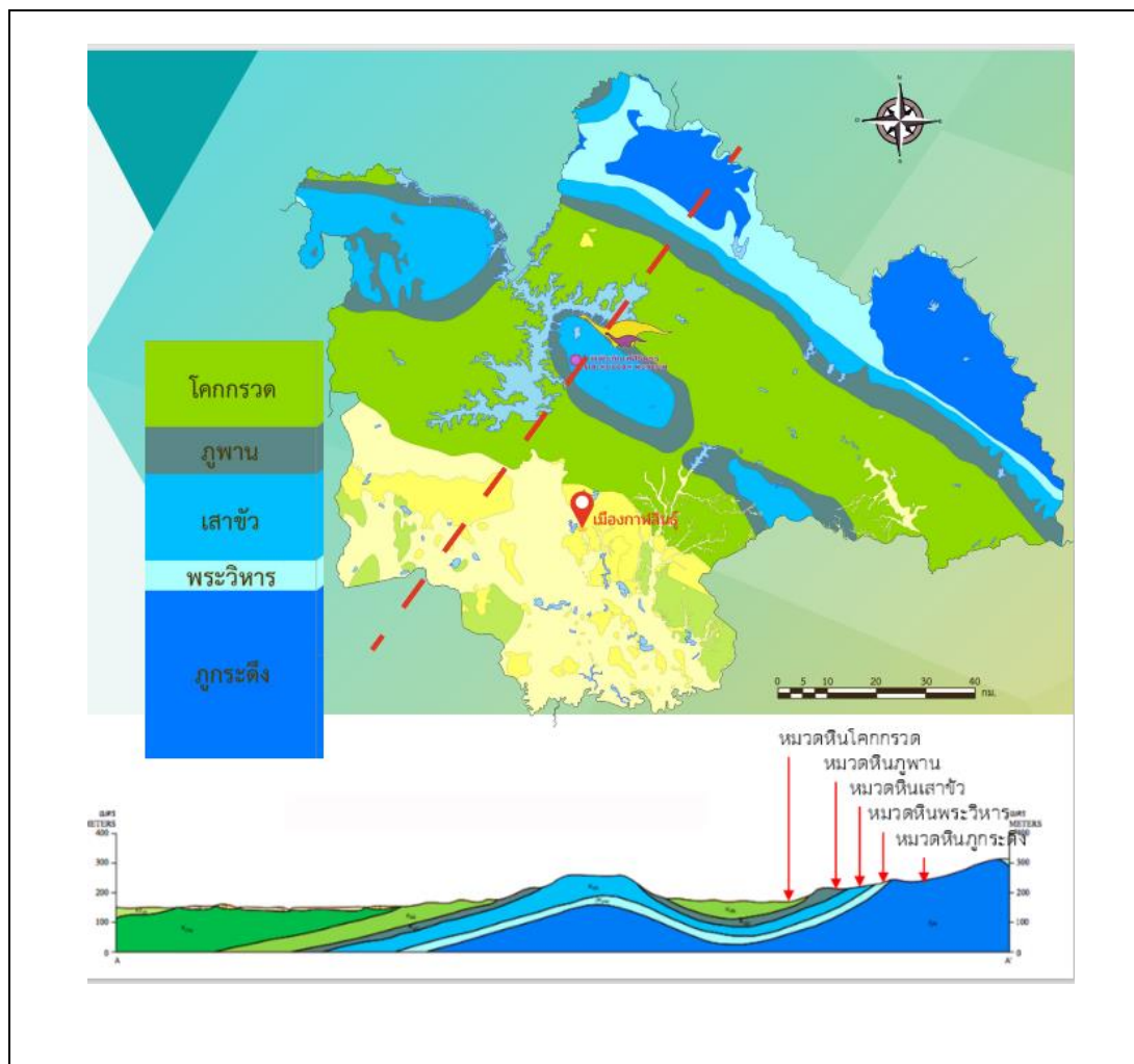
รูปที่ ๒.๑๔ ธรณีวิทยาของแหล่งไดโนเสาร์ภูกุ่มข้าว (พรเพ็ญ จันทสิทธิ์, ๒๕๖๖)
